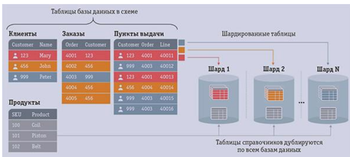
Рис. 2. Пример шардирования семейства таблиц базы данных
