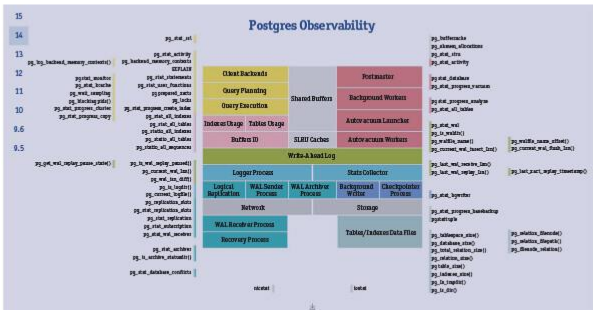
Рис. 3. Postgres Observability
