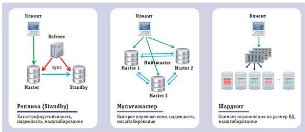
Рис. 1. Механизмы обеспечения архитектуры высокой надежности
